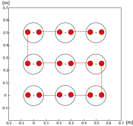
Figure 4 : Disposition des puits utilisée pour le cas de validation
