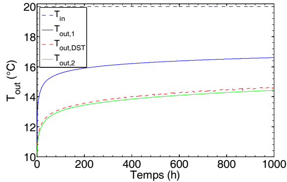
Figure 3 : Comparaison entre les modèles NBiS (2) et DST
