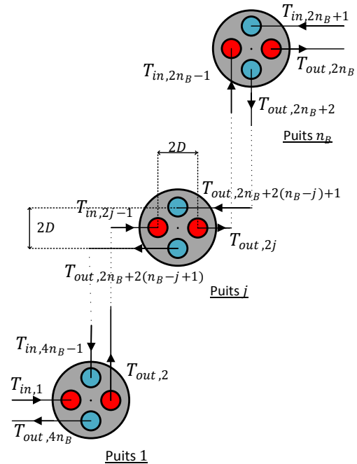
Figure 6 : Circuit de puits à 4 tuyaux et 2 circuits
