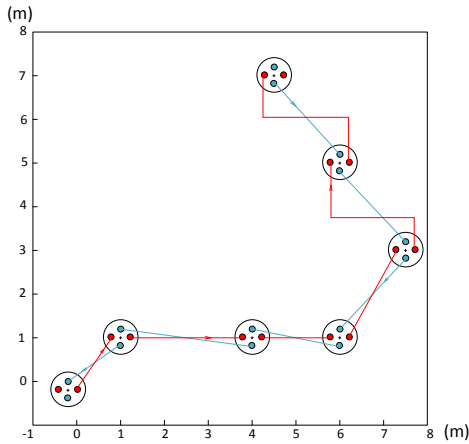
Figure 8 : Circuit de puits à 4 tuyaux avec deux circuits indépendants
