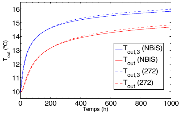
Figure 5 : Comparaison entre le NBiS et le Type 272
