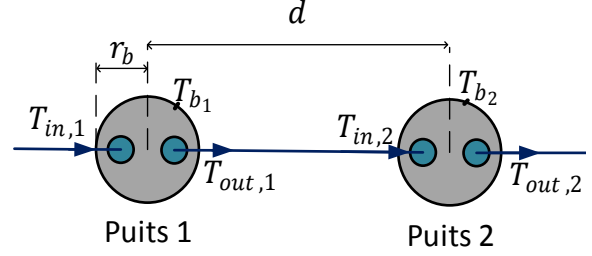
Figure 2 : Coupe A-A de la Figure 1
