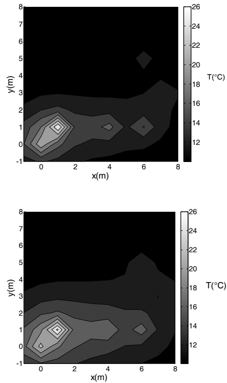
Figure 9 : Isothermes selon les modèle NBiS (haut) et Type 272 (bas)
