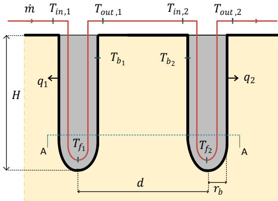
Figure 1: Schéma du problème à deux puits en série
